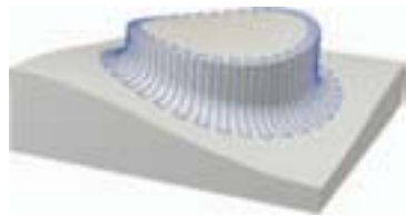
Radiales Schichten mit kreisförmiger An- und Abfahrbewegung
